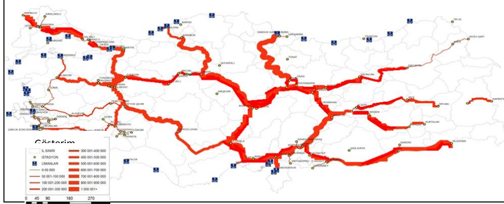
Şekil 2.3.4.1 Demiryolu hatlarına göre yük yoğunluk haritası
